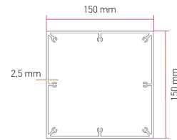
עמוד 150 × 150 mm
